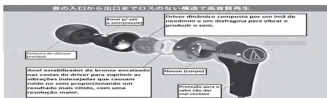
Figura 04 - Elementos básicos de fones de ouvidos
