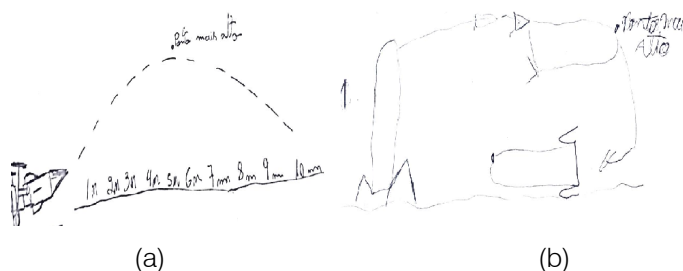
Figura 3 - Desenho da trajetória do foguete PET para um observador fixo na quadra. (a) desenho classificado como QS; (b) desenho classificado como NS
